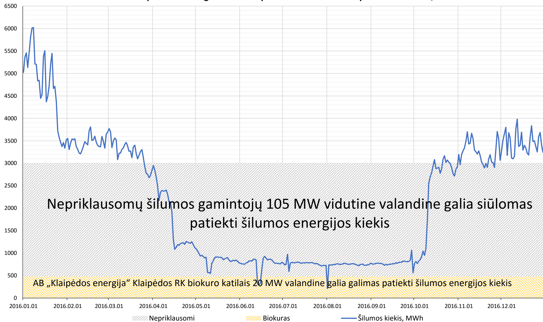
Klaipėdos m. integruoto tinklo paros vidutinis šilumos poreikis 2016 m. , MWh
