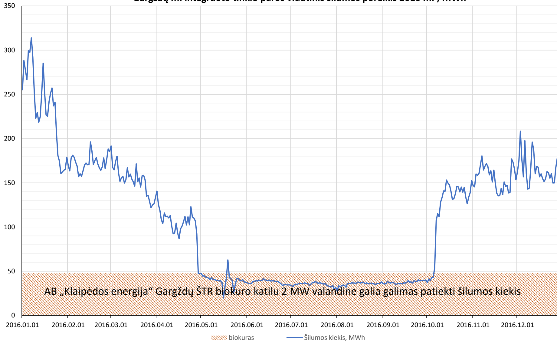
Gargždų m. integruoto tinklo paros vidutinis šilumos poreikis 2016 m. , MWh
